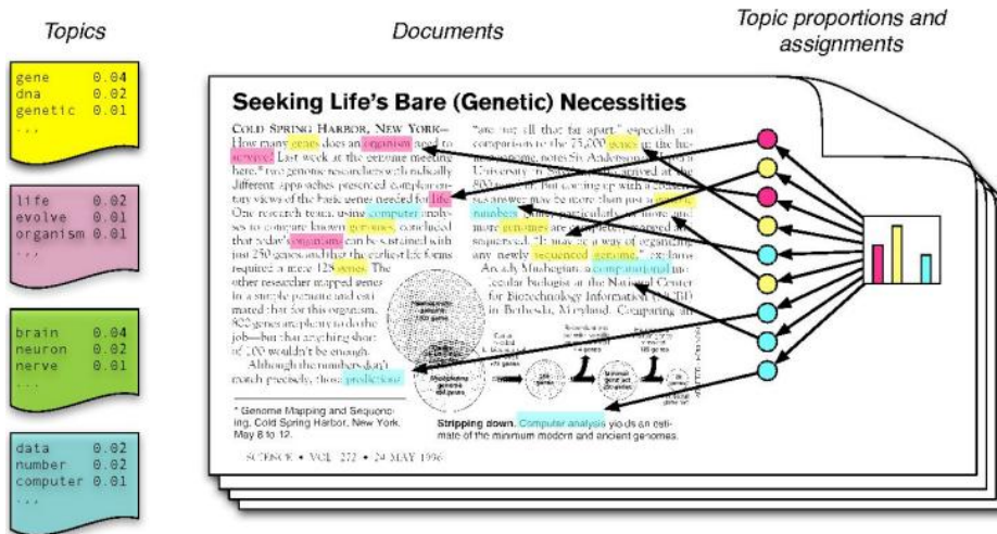
Gambar 4.1 Latent Dirichlet Allocation (LDA)
