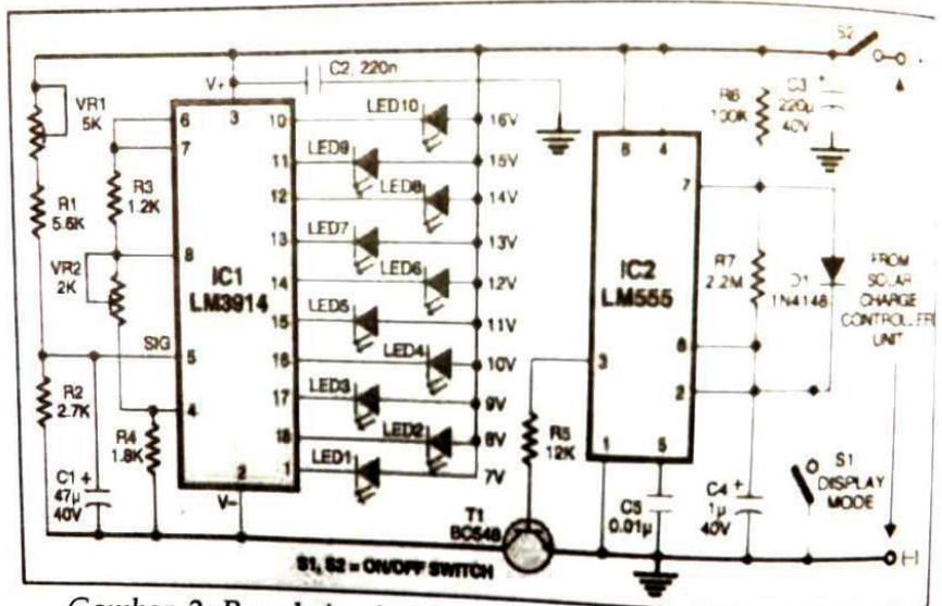
Gambar 3.4 Rangkaian elektronik indikator pengisian baterai tenaga surya
