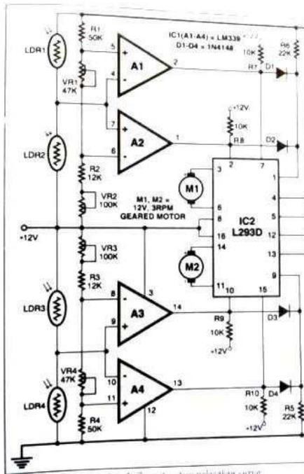
Gambar 3.3 Rangkaian elektronik sistem pelacakan surya
